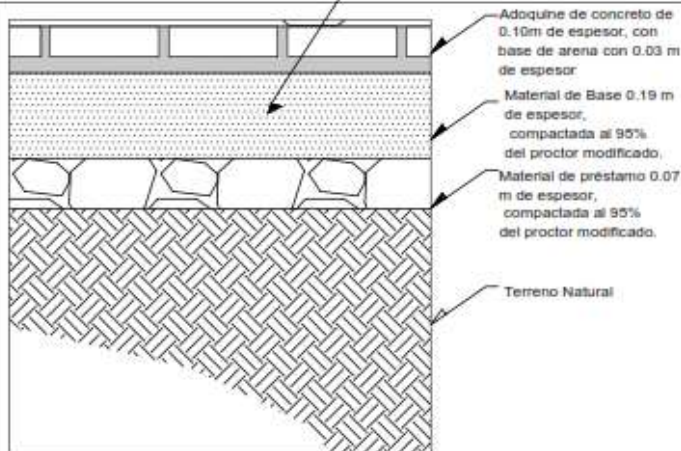
Detalle de superficie de rodamiento Sin escala
